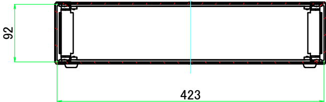
B-B ( 1 : 6 )
